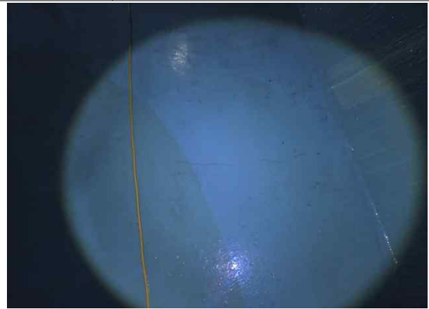
손상내용 1지 바닥슬래브 균열 손상원인 건조수축
